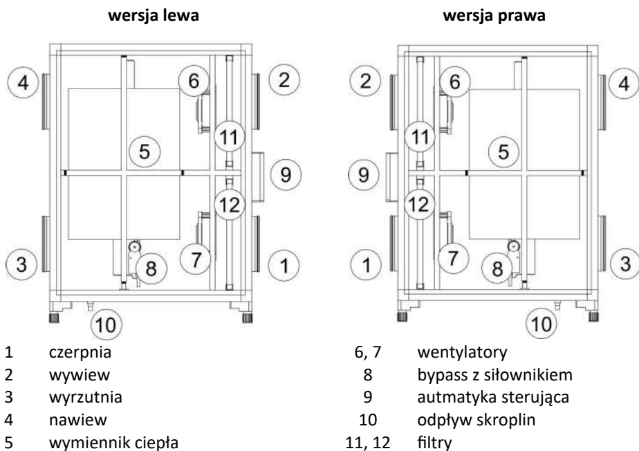
Rys. 1b Schemat budowy centrali Nikol SMART PRO z wyszczególnieniem części składowych w wykonaniu prawym i lewym.
