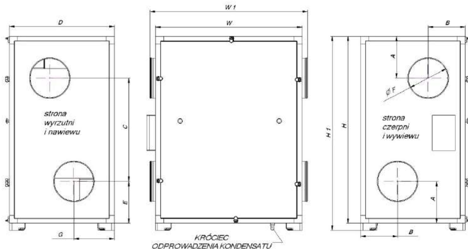
Rys. 1a Wymiary central Nikol SMART PRO
